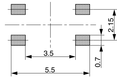
P.C.B LAND DIMENSION
