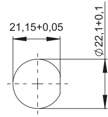
Bohrplan
