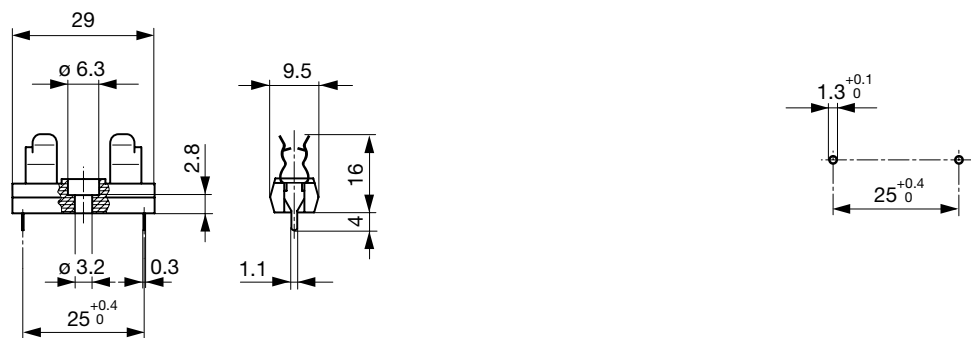
Bohrplan
