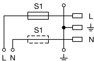
Gerätestecker mit Sicherungshalter (5 x 20 mm)
