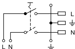
Gerätestecker mit Netzschalter
