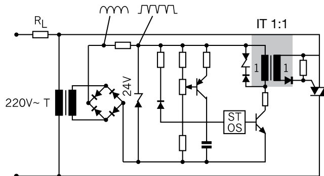
Triac-Phasenanschnittsteuerung
