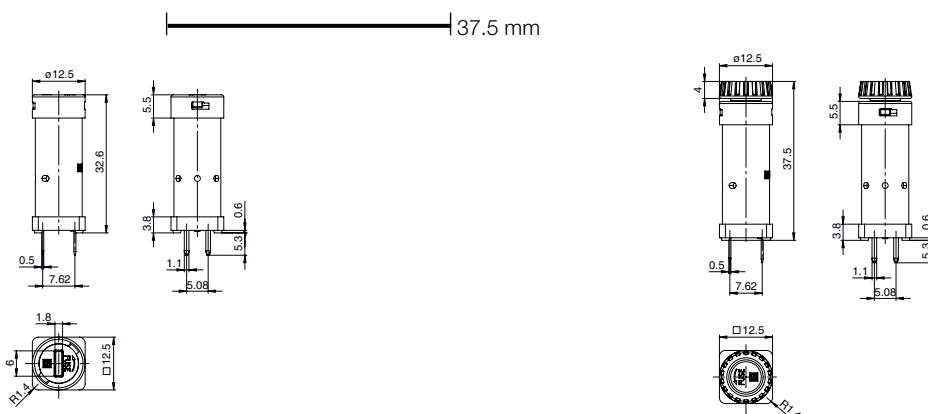
Variante Fingergrip 3101.0045
