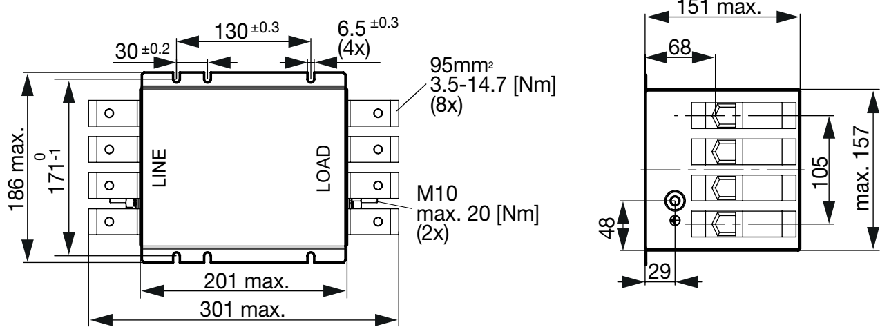
Gehäuse 5D-95
