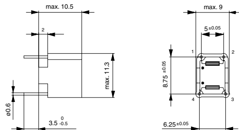
Gehäuse 48-2
