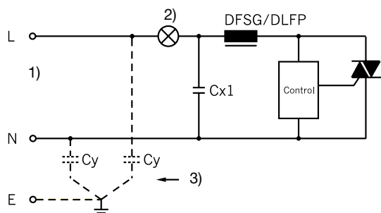
Entstörung bei ohmscher Last, < 10 A, z.B. Dimmerschaltung (DFSGI)
