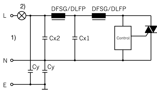
Entstörung bei ohmscher Last, 2-stufig
