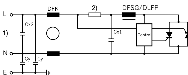
Entstörung einer ohmschen Last, 2-stufig
