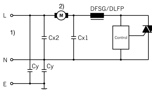
Entstörung bei induktiver Last
