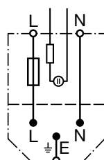
Version mit Anzeigelampe
