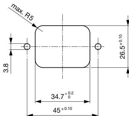
Plattenausschnitt und Bohrdiagramm
